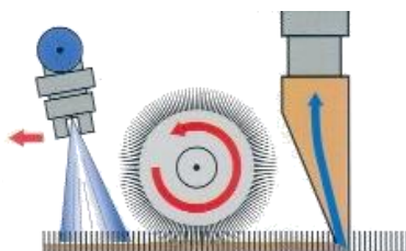
Sistema ad iniezione-estrazione con spazzola rotante
